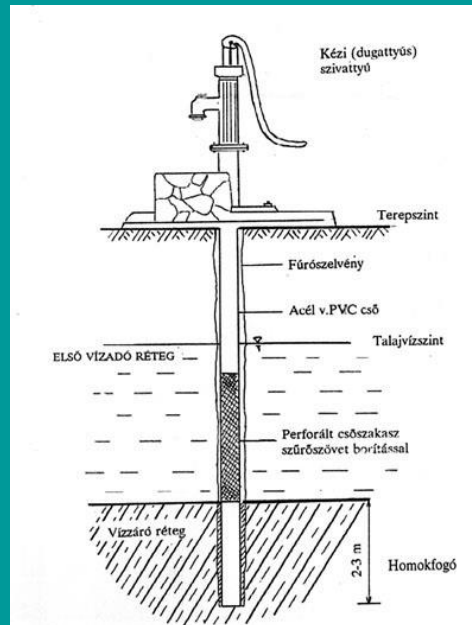
Talajvízre telepített fűrész kút Gerencsér Á. nyomán [1.]
