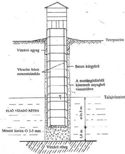
Normál kivitelű ásott kút Gerencsér Á. nyomán [1.]
